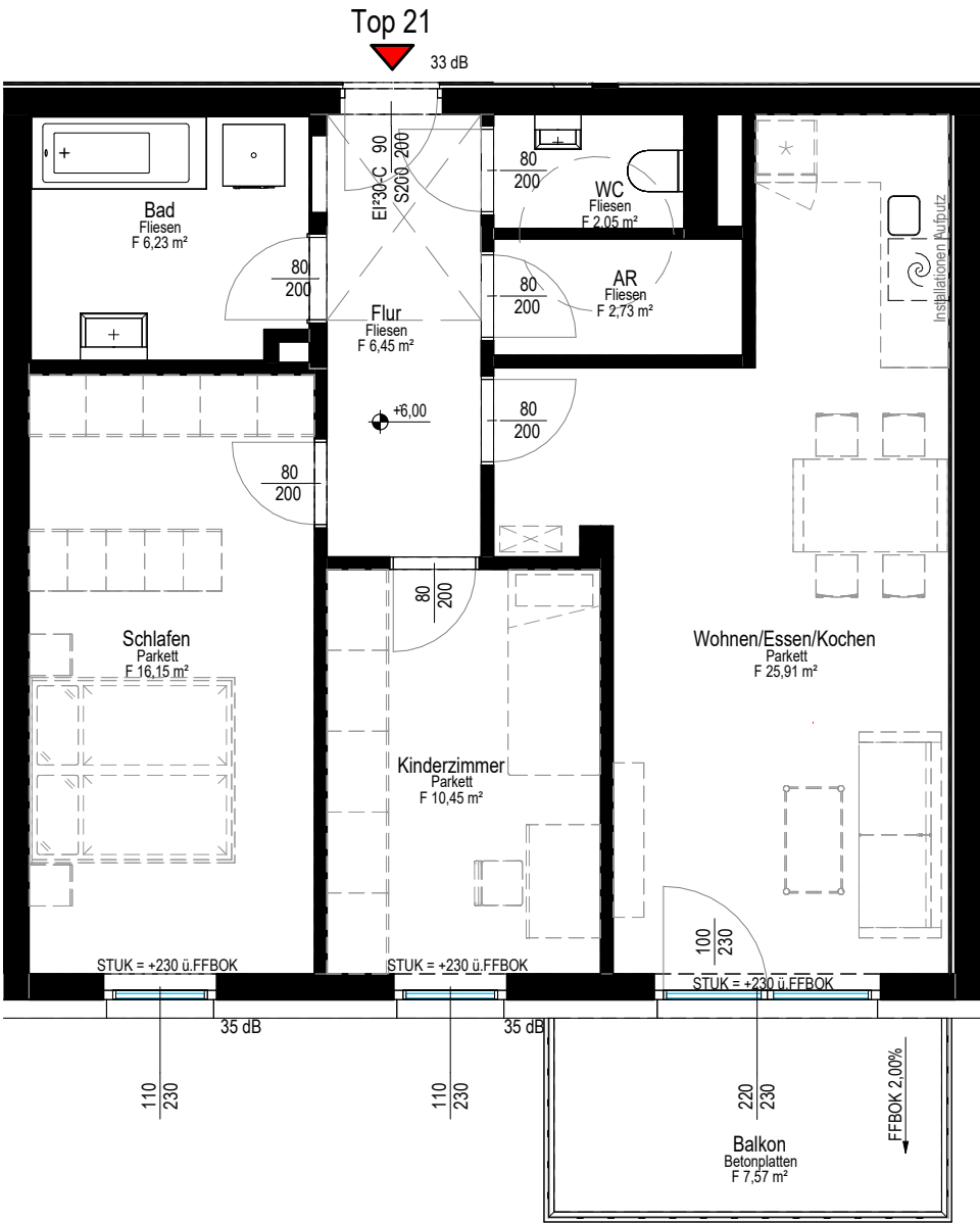
Grundriss M 1:75
