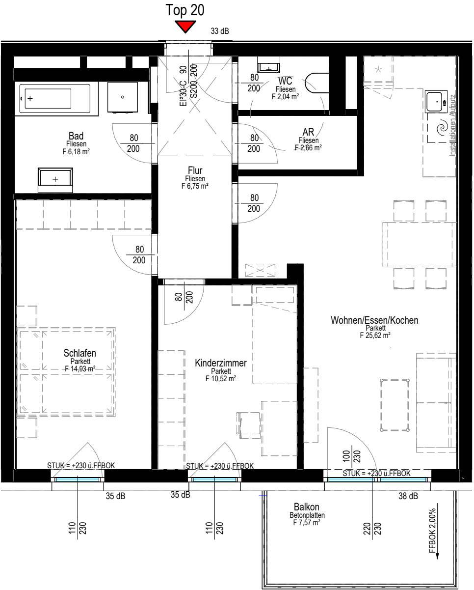
Grundriss M 1:75
