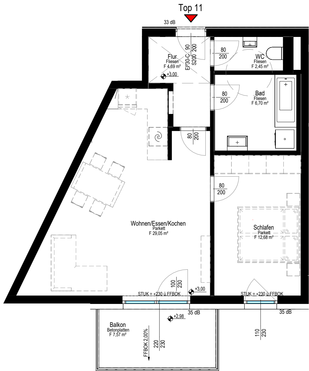
Grundriss M 1:75
