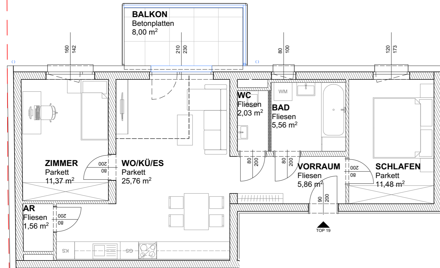
GRUNDRISS | M 1:75
