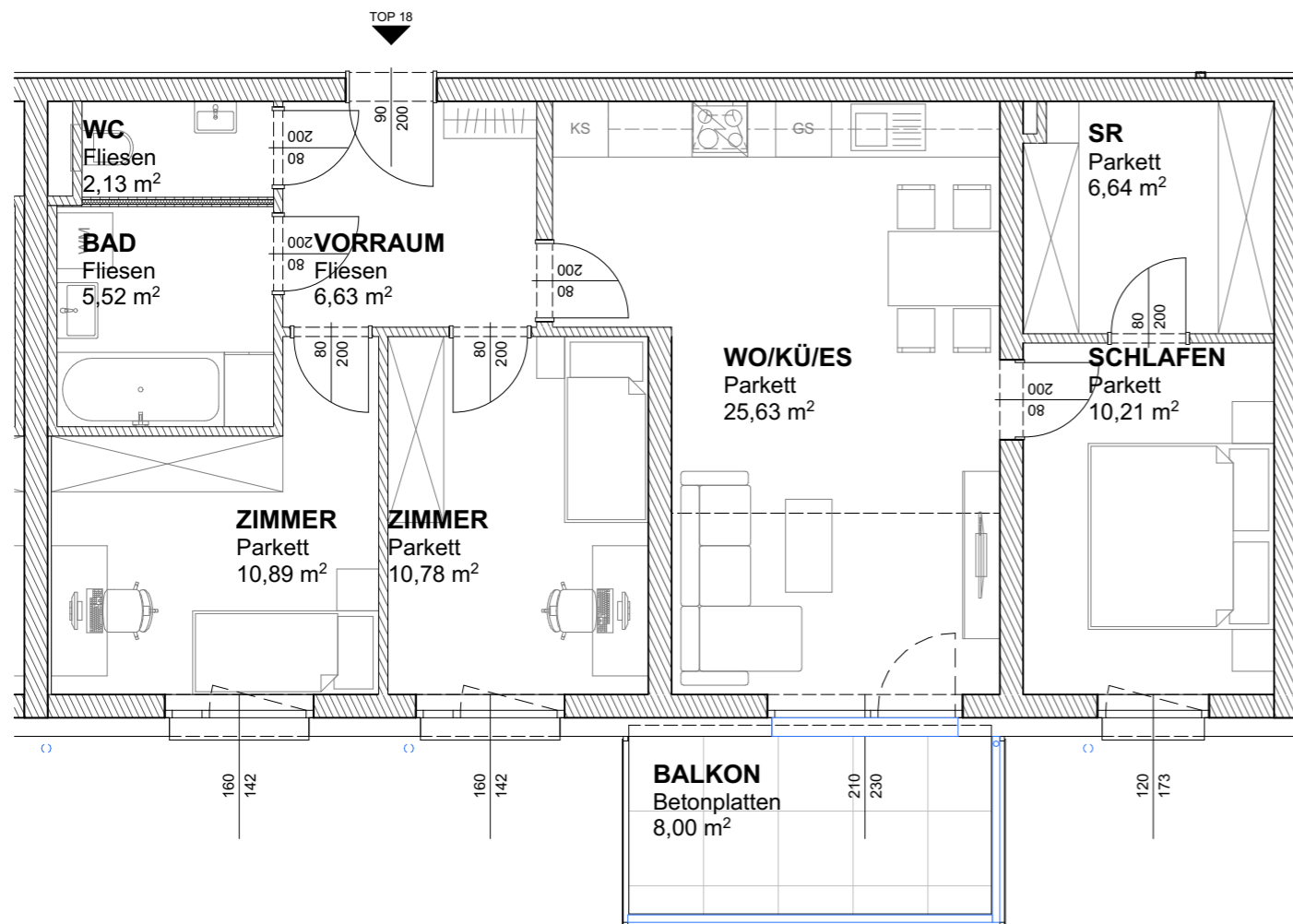
GRUNDRISS | M 1:75
