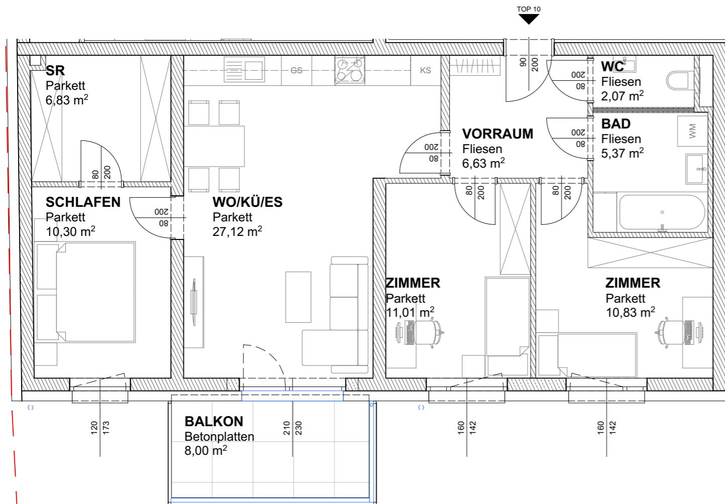
GRUNDRISS | M 1:75
