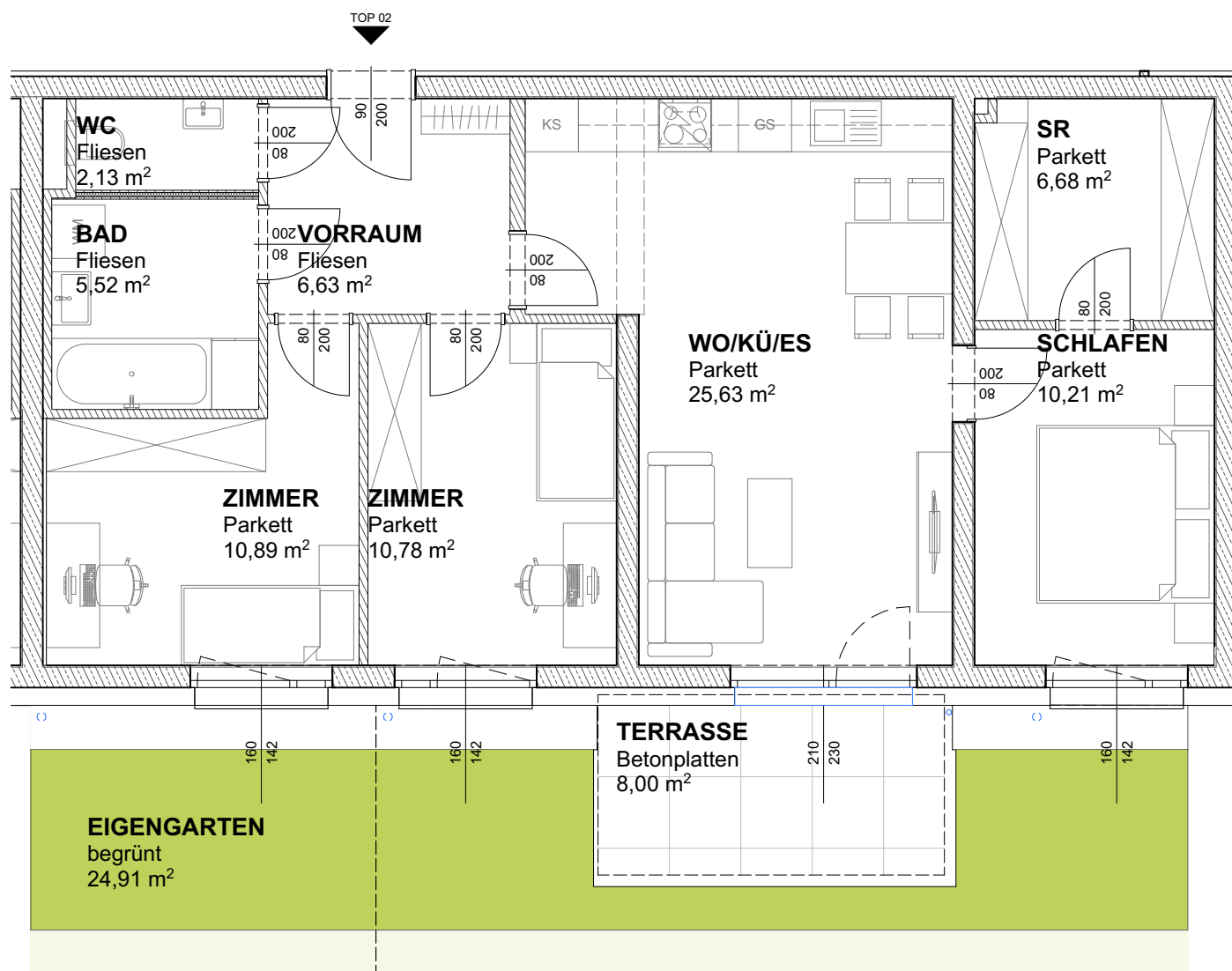
GRUNDRISS | M 1:75
