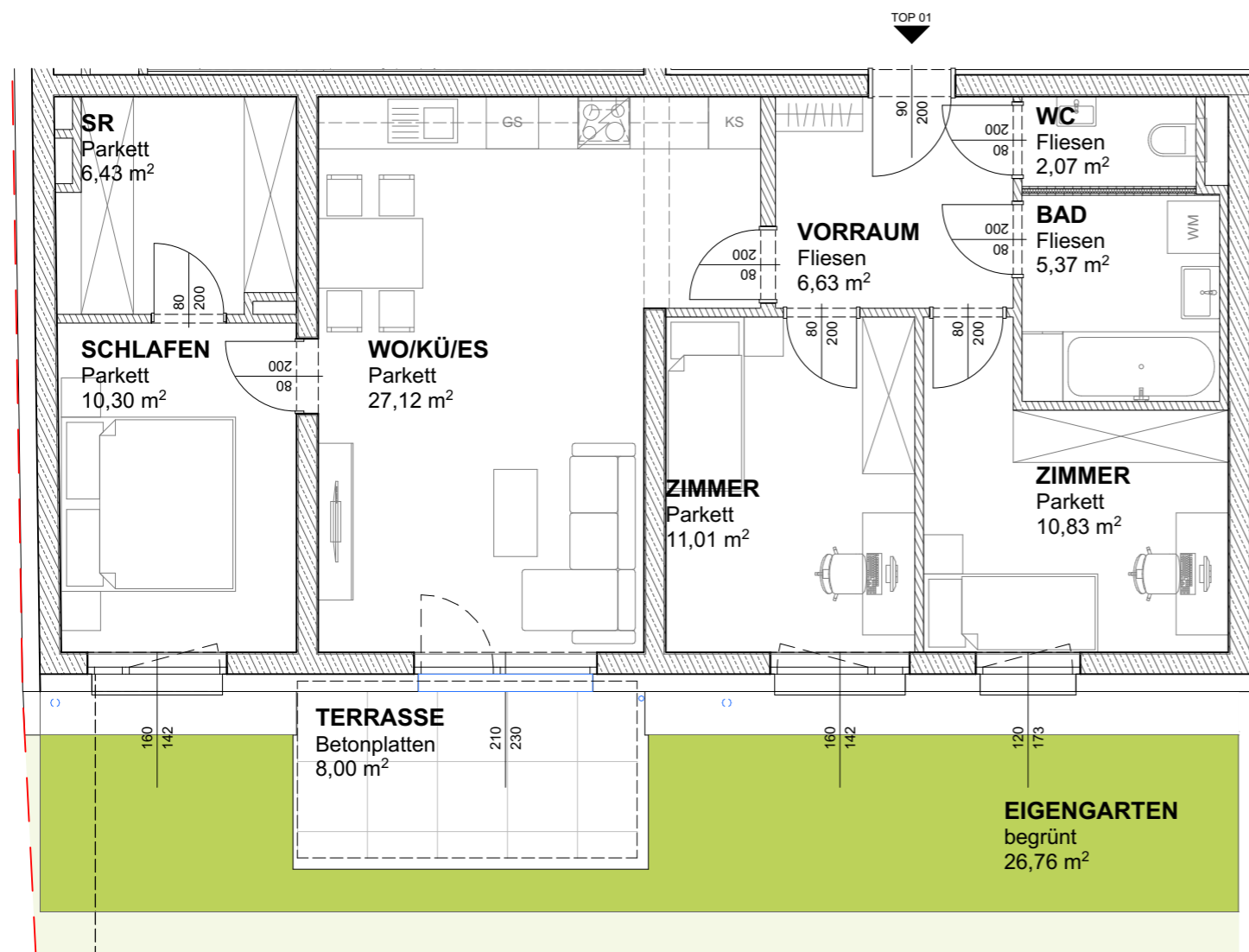
GRUNDRISS | M 1:75
