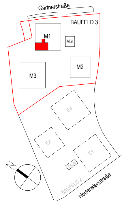
ÜBERSICHTSPLAN
